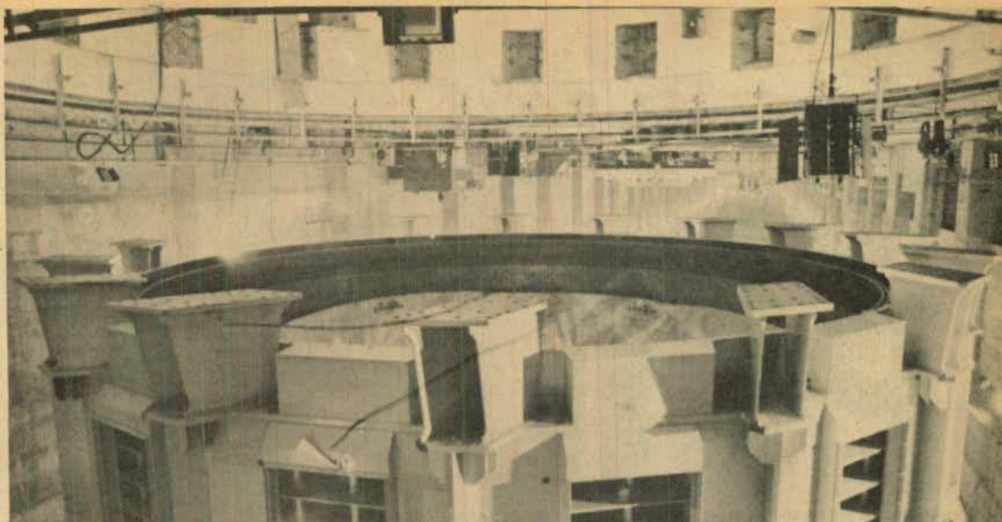
Lentamente, o estator desce à sua base definitiva no poço da Unidade 7
